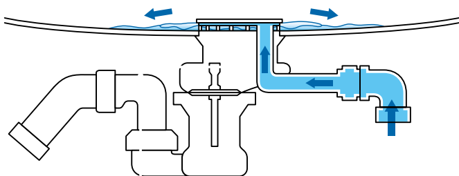
L'entrata è dotata di valvola di ritegno integrata
